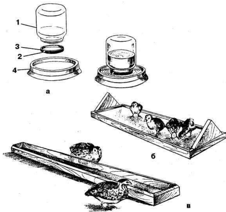
Рис. 28. Оборудование для молодняка раннего возраста: а — поилка вакуумного типа: 1 — емкость для воды; 2 — отверстие для вытекания воды; 3 — подставка; 4 — миска; б — кормушка-противень; в — кормушка желобковая
